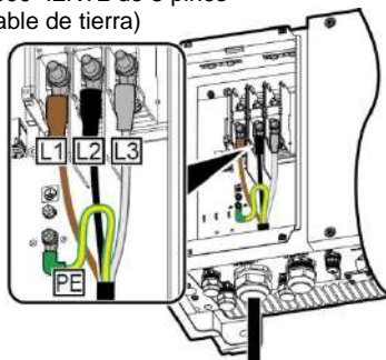
d. SUN2000-42KTL de 4 pines (con cable de tierra pero sin conductor neutro)
