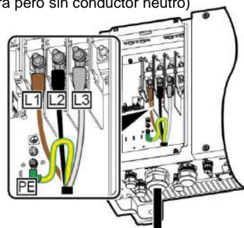
f. SUN2000-33KTL-A/36KTL (con cable de tierra pero sin conductor neutro)
