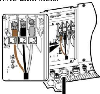
e. SUN2000-33KTL-A/36KTL (sin cable de tierra ni conductor neutro)
