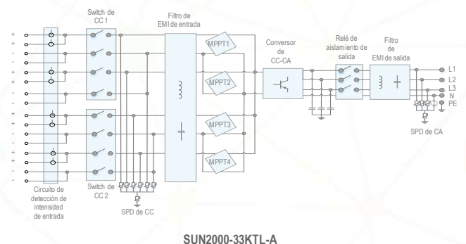
Esquema eléctrico
