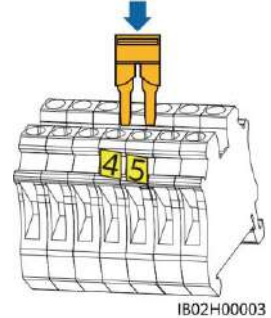
Terminal de CA para redes eléctricas (X2) (monofásico/trifásico)
